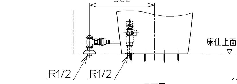
正面図
